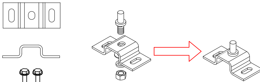
Bottom Hinges
