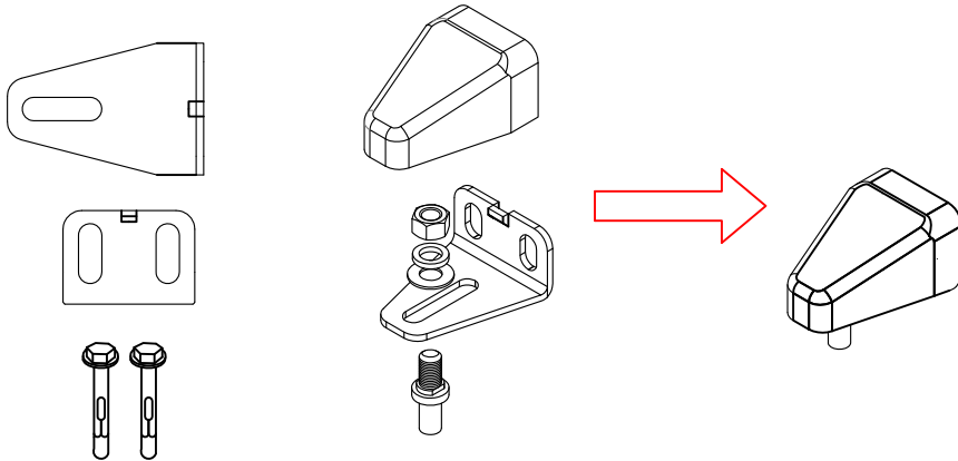
Top Hinges
